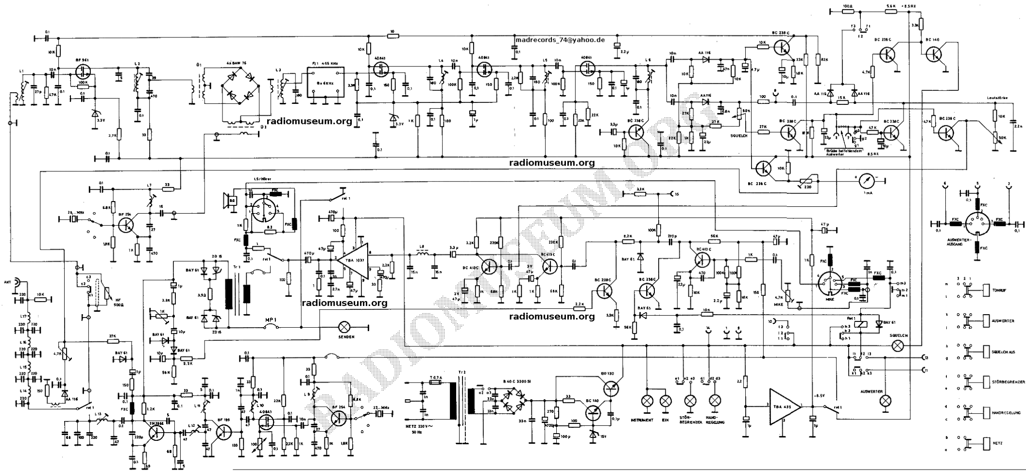
Schaltplan SE 411
